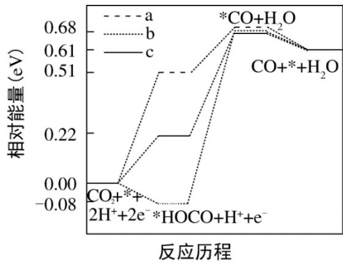
(a) \text{CO}_2 电还原为 CO
